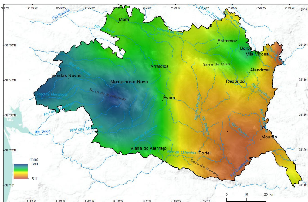
Figura 5. Precipitação média anual no Alentejo Central (1971-2015)
