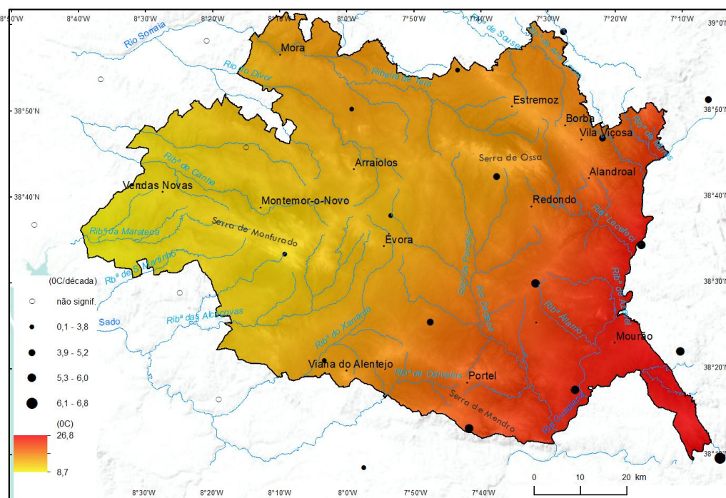
Figura 4. Número médio anual de dias muito quentes e tendência recente no Alentejo Central (1971-2015)
