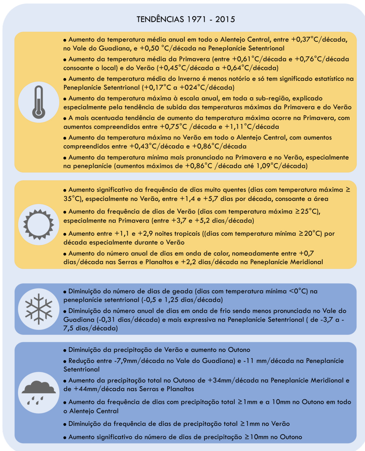
Figura 6. Principais tendências observadas no Alentejo Central (1971-2015)
