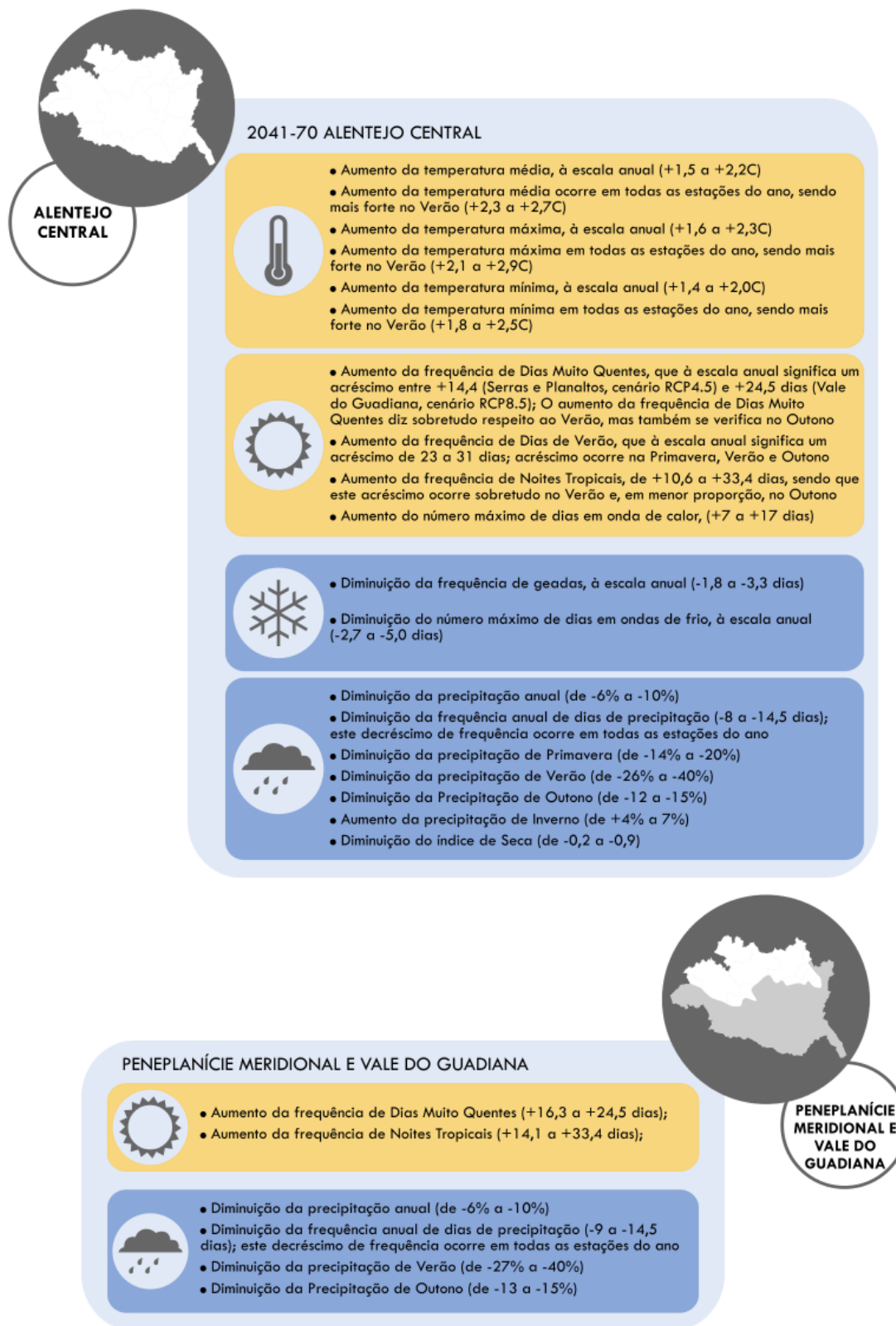
Figura 7. Cenários Climáticos para o Alentejo Central (2041-2070)
