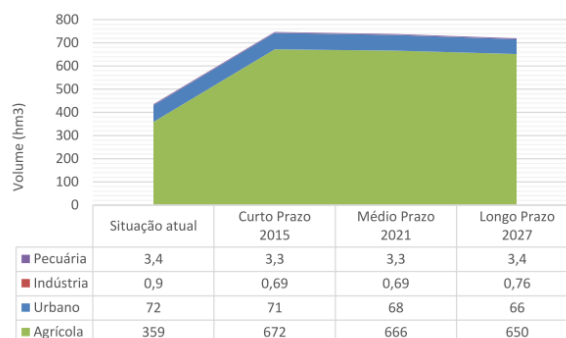
Figura 64 – Projeções de volume captado para o cenário business as usual na Região Hidrográfica 7 (PGRH7 2016c)
