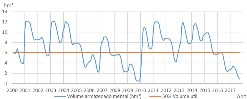
Figura 80. Volume armazenado mensalmente na albufeira do Divor no período 2000-2017
