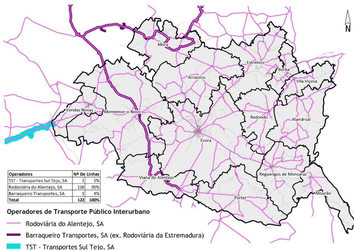
Figura 59. Oferta do transporte público rodoviário no Alentejo Central
