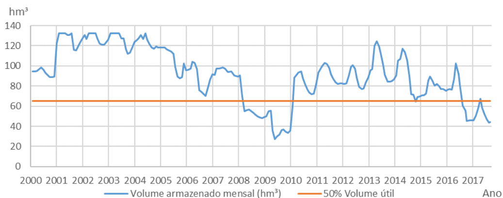
Figura 78. Volume mensalmente armazenado na albufeira do Alvito no período 2000-2017
